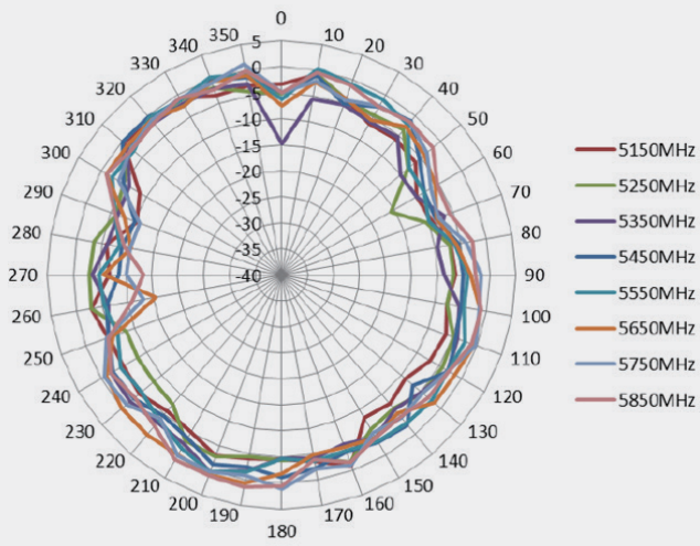
5G (PHI=0)
