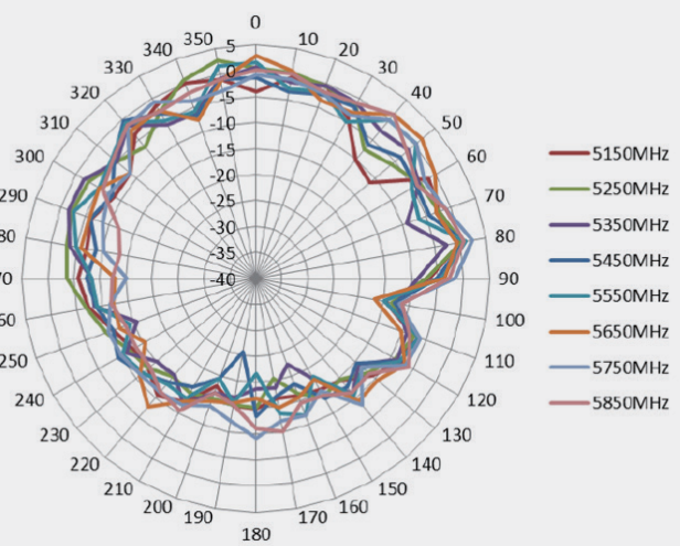
5G (PHI=90)
