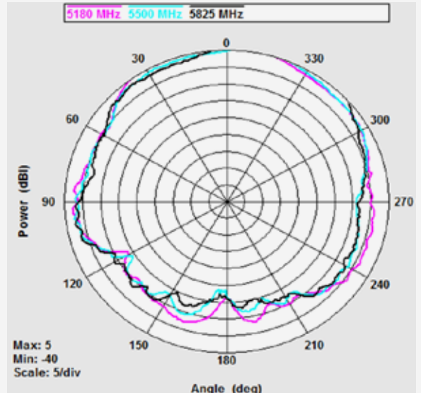
5G (PHI=90)
